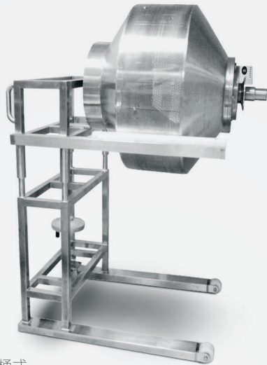
換桶式 Change pan type
